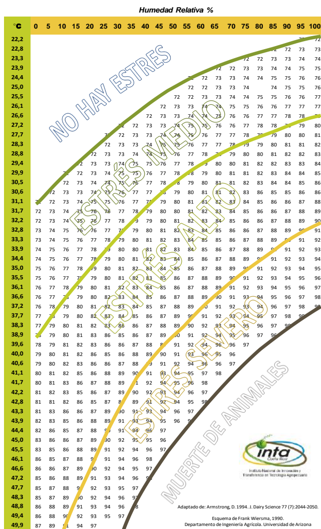
ESQUEMA PARA DETERMINAR ESTRÉS TÉRMICO EN VACAS LECHERAS
