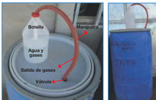
Figura 34. Diagrama del estañón, funcionamiento y posicionamiento de manguera.
